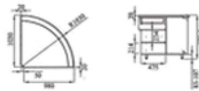
BBCAI90 - BALCÃO BAIXO CALADE ÂNGULO INTERNO 90°
