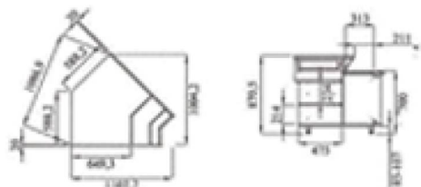
ECCXAI45 - BALCÃO CALADE CAIXA ÂNGULO INTERNO 45°
