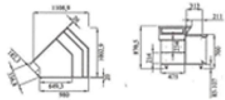
ECCXAI45 - BALCÃO CALADE CAIXA ÂNGULO INTERNO 45°
