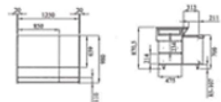
ECCXAE45 - BALCÃO CALADE CAIXA ÂNGULO EXTERNO 45°
