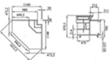
ECCXAI90 - BALCÃO CALADE CAIXA ÂNGULO INTERNO 90°
