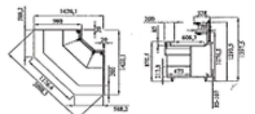
VCNAE90 - VITRINA CALADE NEUTRA ÂNGULO EXTERNO 90°
